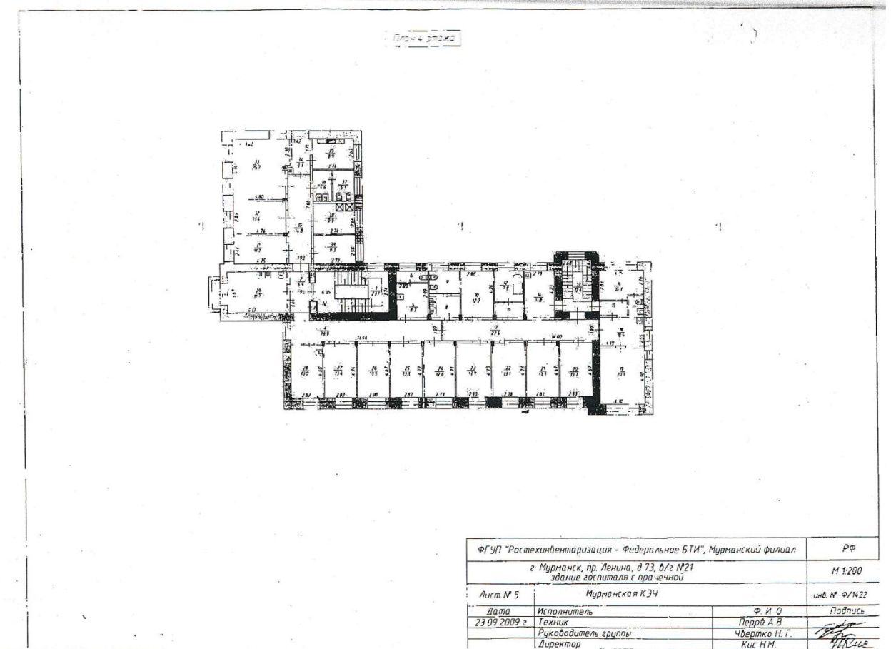
Изображение 11. План 4-го этажа. Технический паспорт 2009 г.
