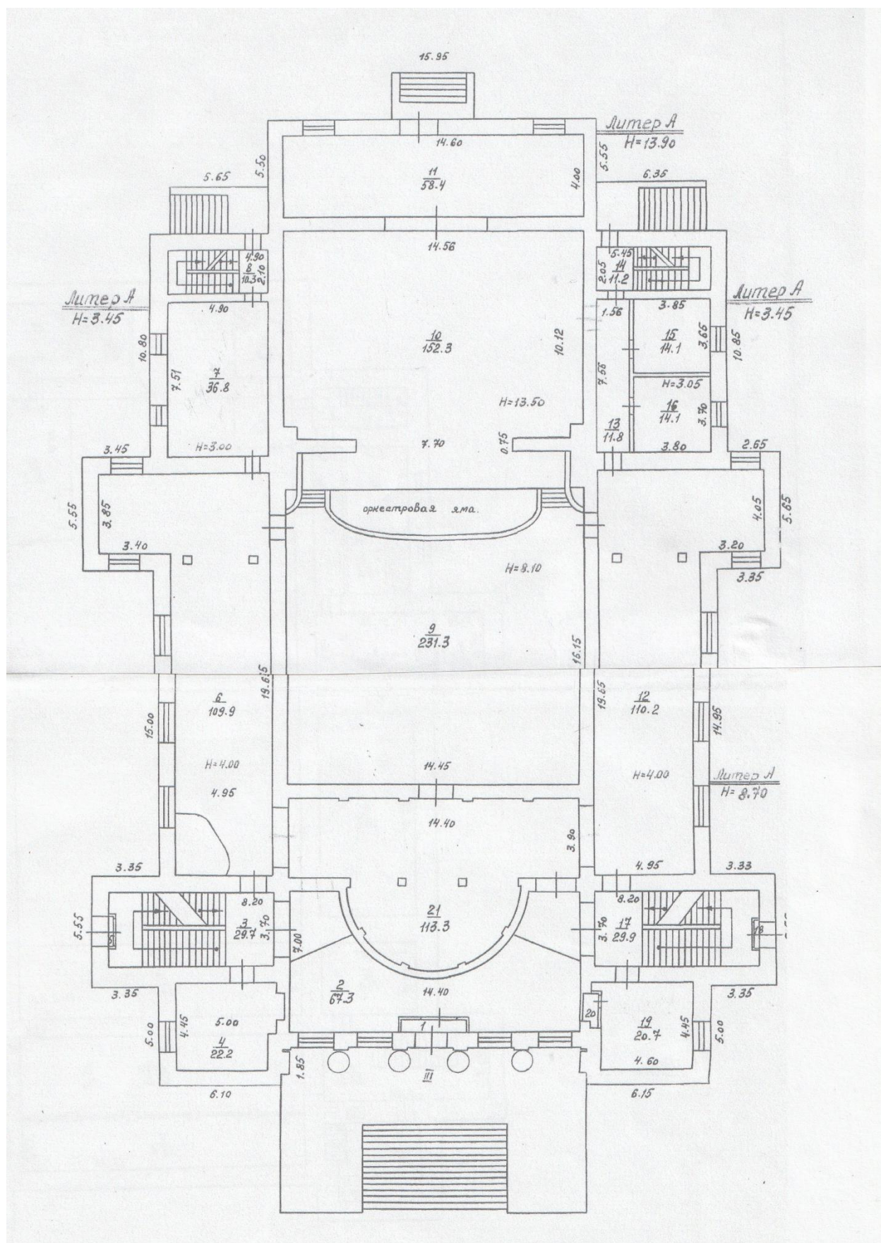
27. Технический паспорт 1986 г. План 1-го этажа.
